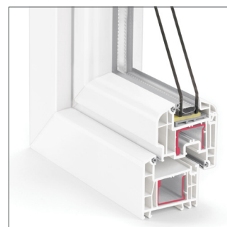
skrzydło zaokrąglone
